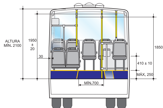
CORTE AB
