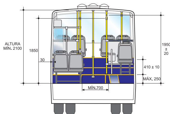
CORTE AB
