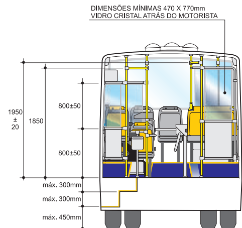
CORTE CD
