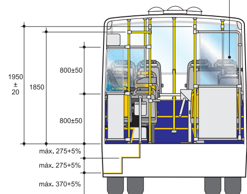
CORTE CD
