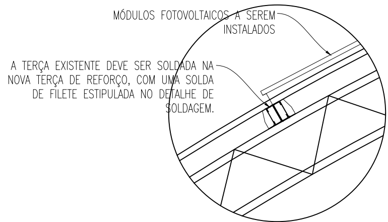
DETALHE TÍPICO DA TERÇA DE REFORÇO ESCALA 1:25
