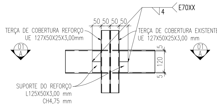
DETALHE TÍPICO DE LIGAÇÃO DA TERÇA DE REFORÇO BANZO UE130X50X3,00 X TERÇA UE127X50X25X3,00 ESCALA 1:10
